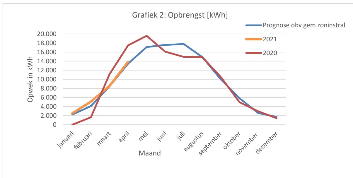
Grafiek 2: Opbrengst ECO installatie in kWh
